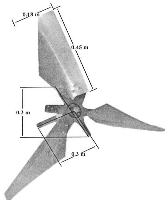
Figure-4. Turbine of VMWT.
