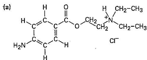
Procaine
