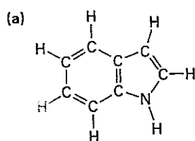
Indole
